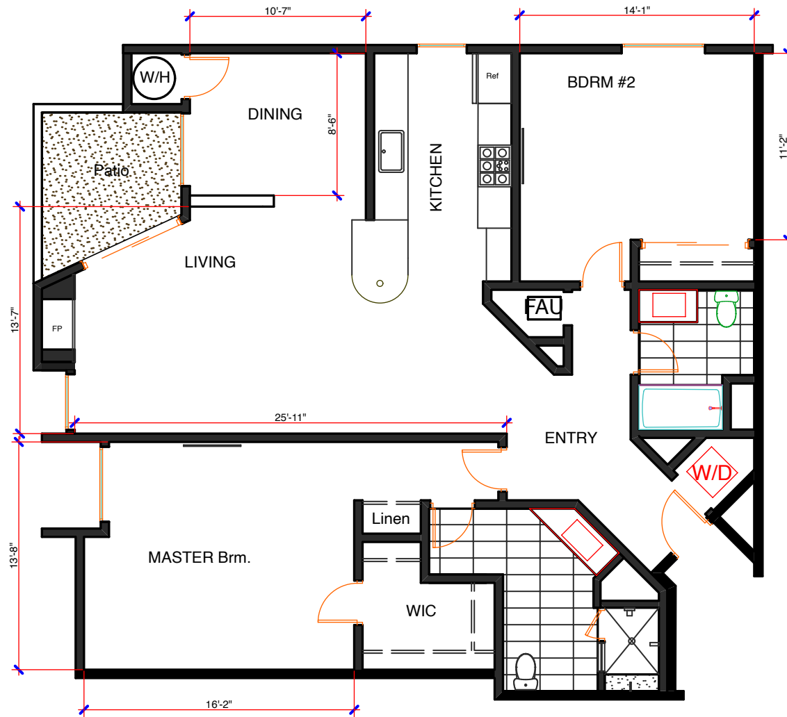
Unit 204 UNIT TYPE 'B'
